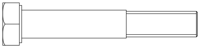
A3 M10X70 Hex Head Bolt Qty.2
